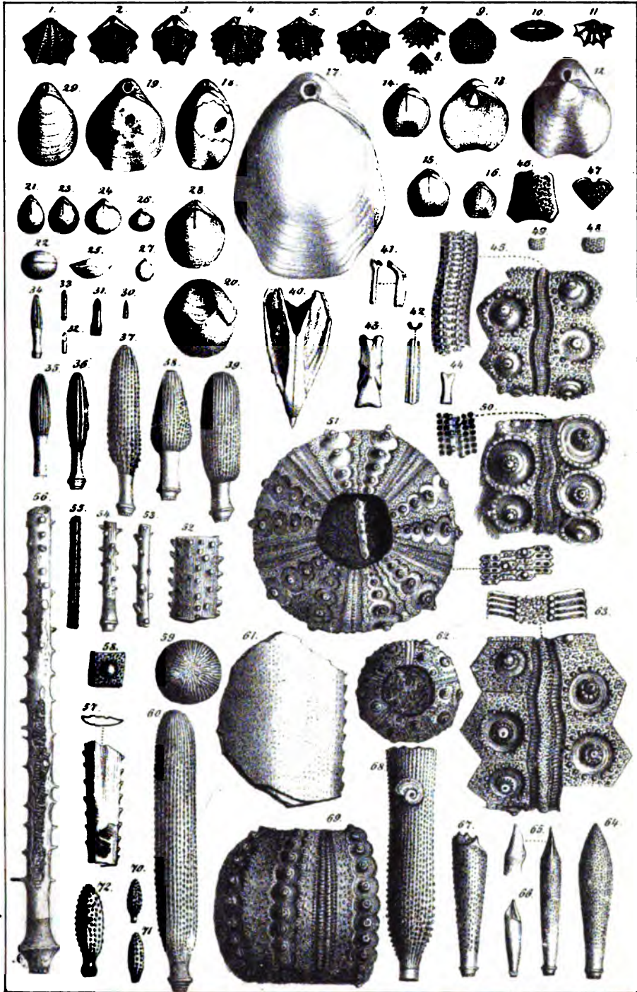
(Jura, Jura.)
